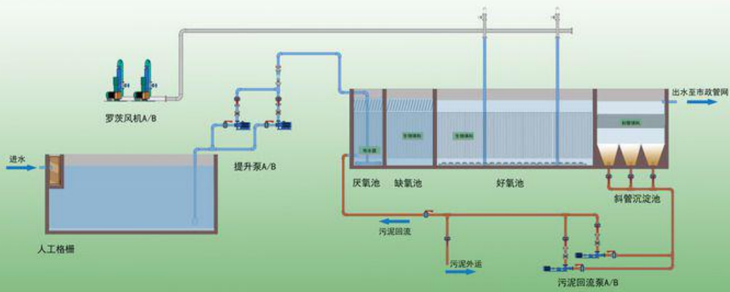
200m 3 /d生活污水处理工艺流程图
